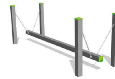
REF M-PS40 POUTRE MOBILE HCL 0,3 m ZI 5,89 x 3,93 m - 21,5 m 2 à partir de 1m40
