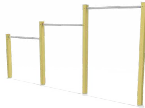
3 à 12 ans REF BF100 BARRES FIXES HCL 1,6 m ZI 6,37 x 3,29 m - 18,5 m 2
